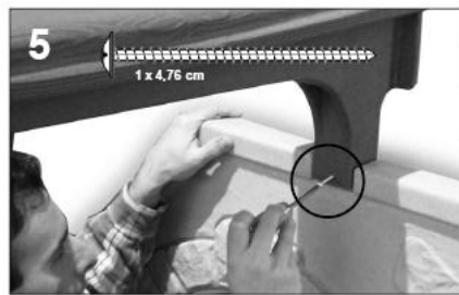
Nasadte hřeben střechy a na přední části přišroubujte.
